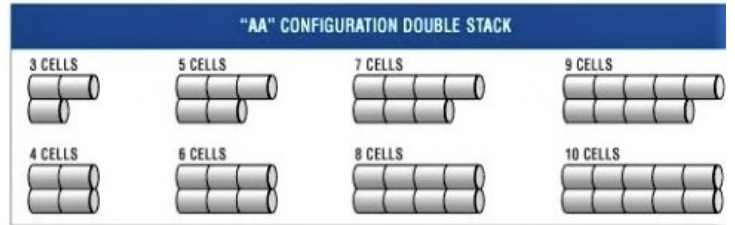
AA - jungimas nuosekliai per dvi eilutes
